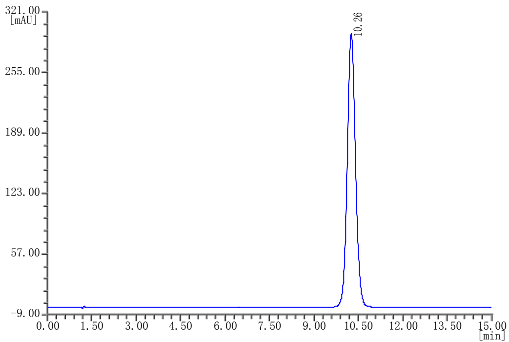
三氯卡班样品的色谱图
